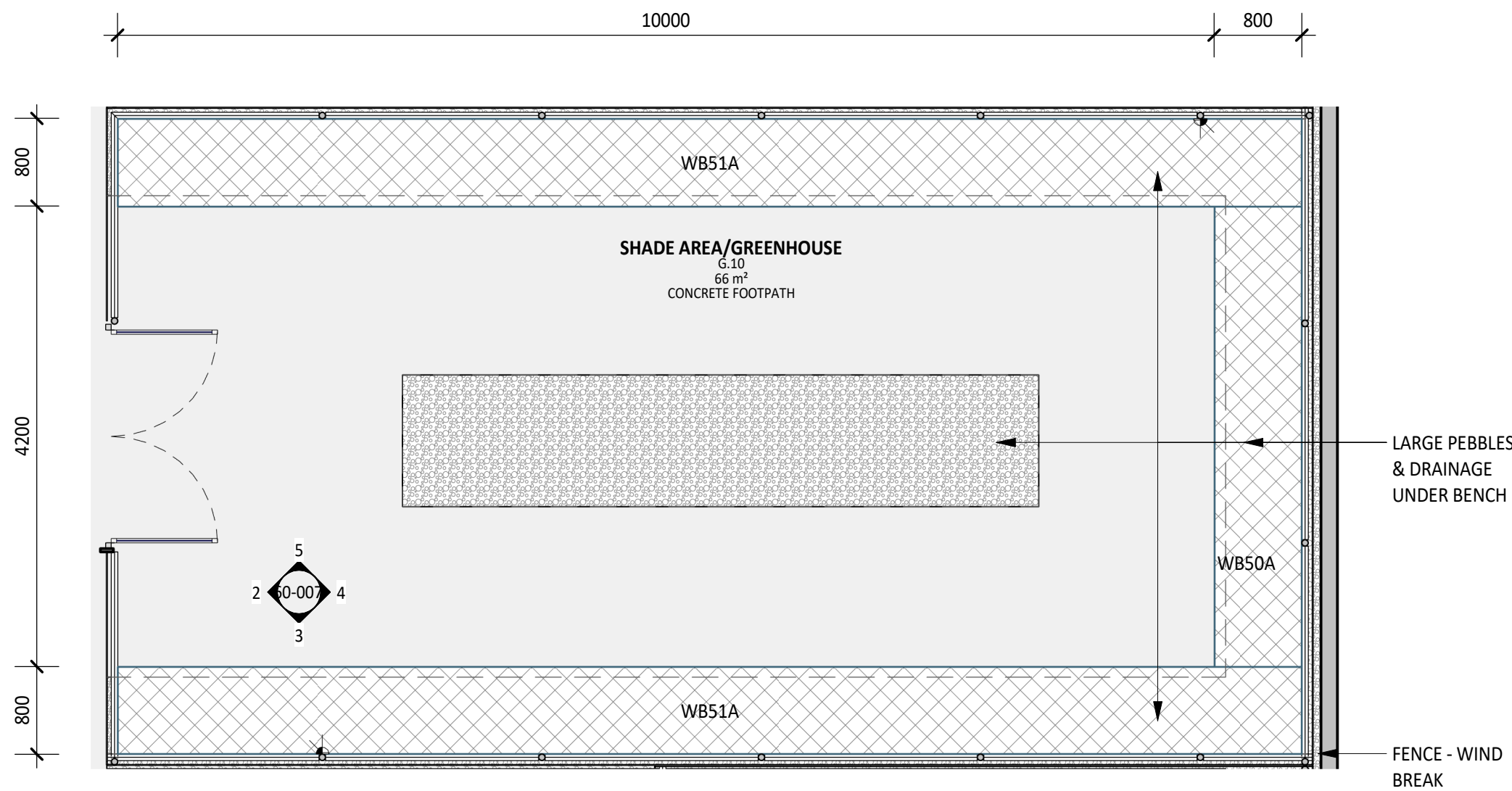
1 PLAN DETAIL 1 : 50
