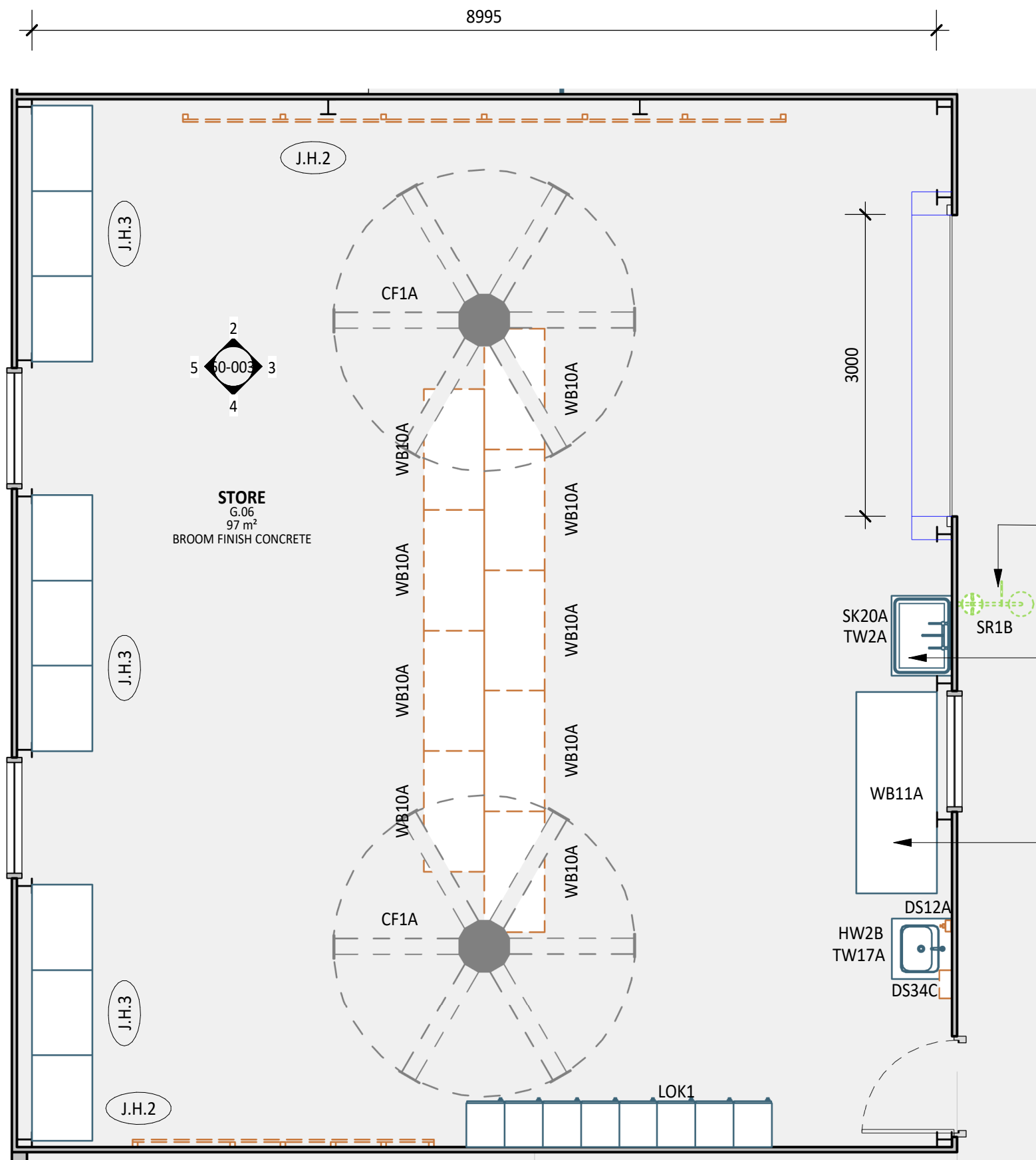
1 PLAN DETAIL 1 : 50
