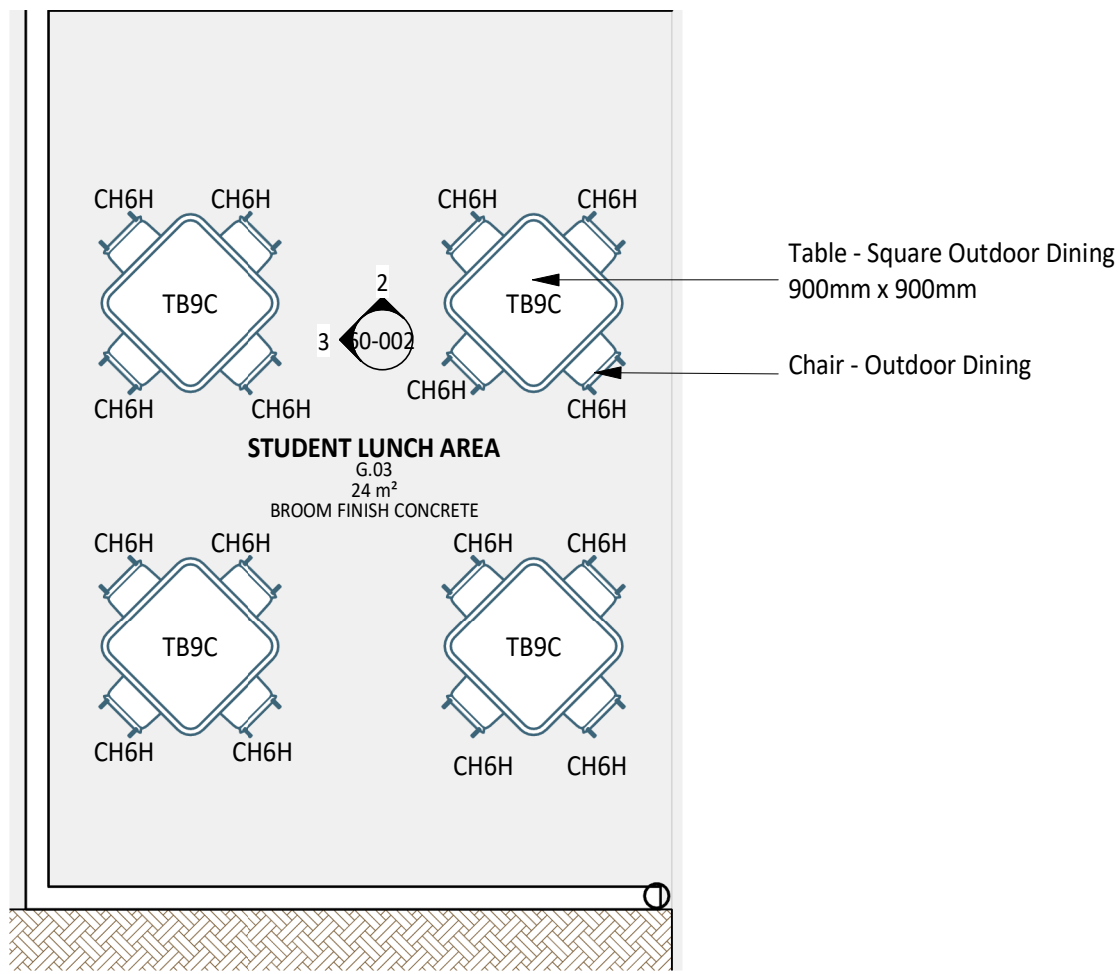
1 PLAN DETAIL 1 : 50
